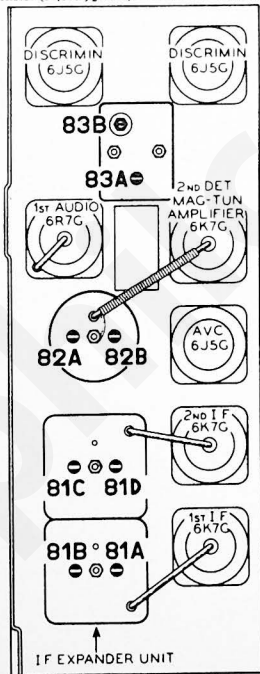
Fig. 7. I. F. Compensators
