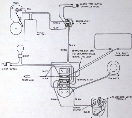
Wiring Diagram—Model H-1335
