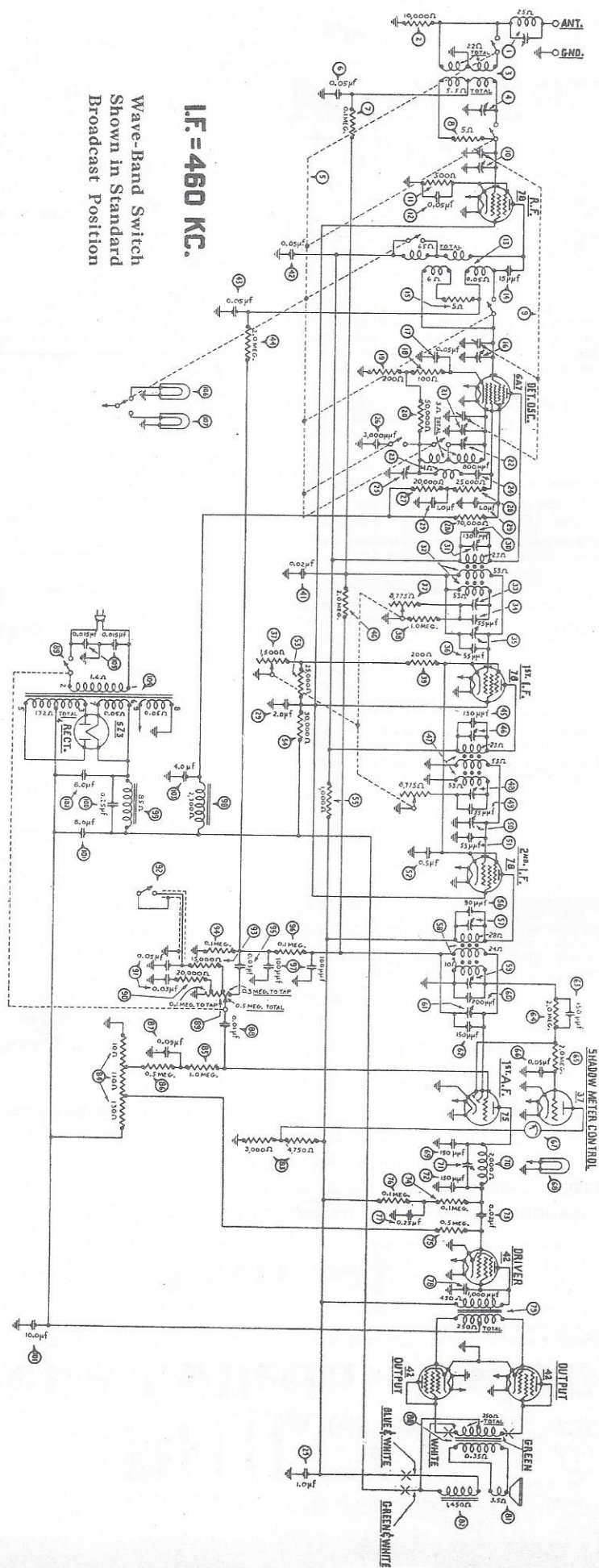
Fig. 2—Model 201 (Code 121) Wiring Diagram
